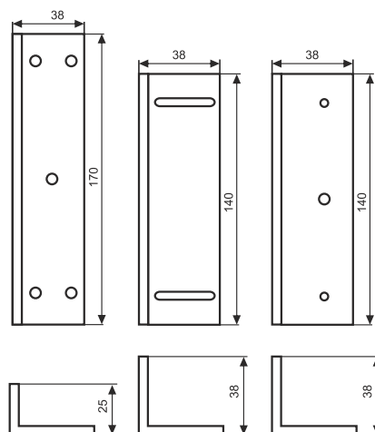
OP 1001M 150 kg
