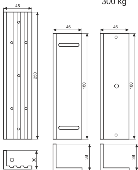
OP 3701M 300 kg
