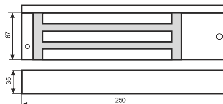
Model 13000M - wersja podstawowa Model 13100M - wersja z przełącznikiem NO/NC i sygnalizacją LED.
